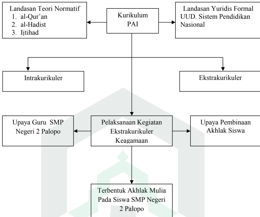
Gambar 2.1 Kerangka Pikir
