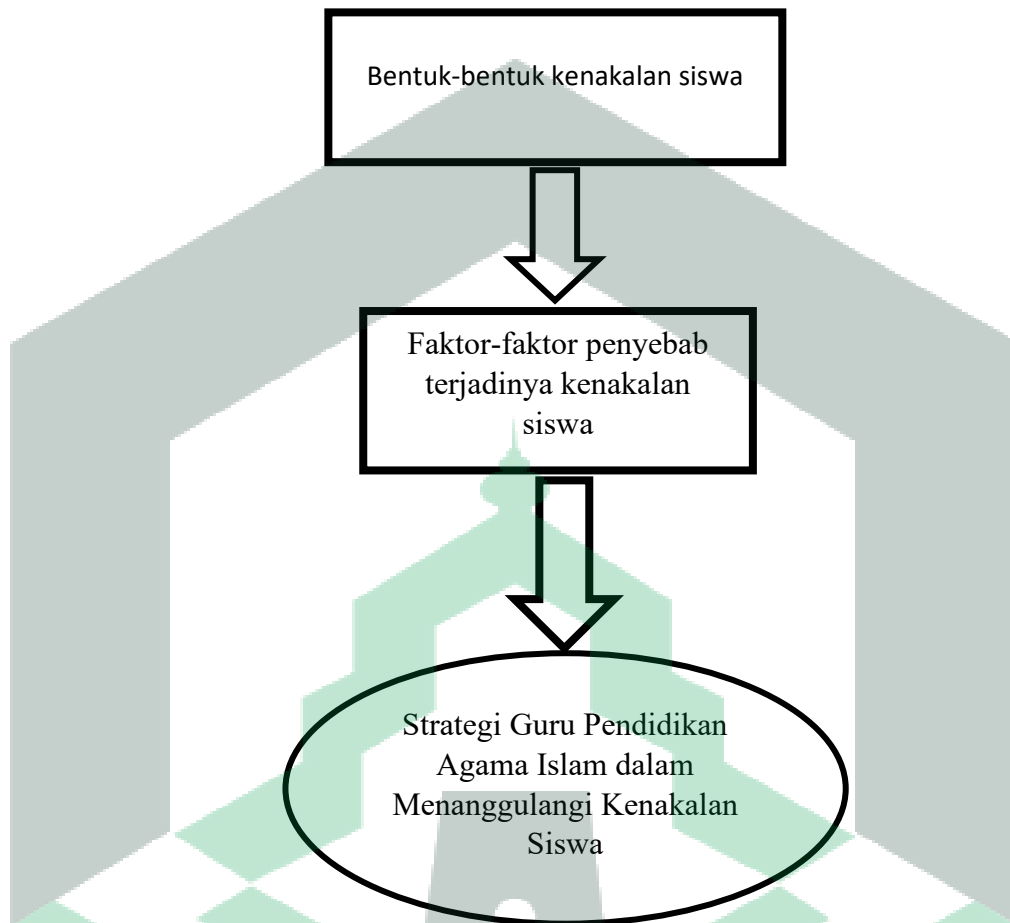
Gambar 2.1 Kerangka Pikir
